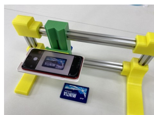
スマホ向け複写台 高さ調整 10cm~20cm
